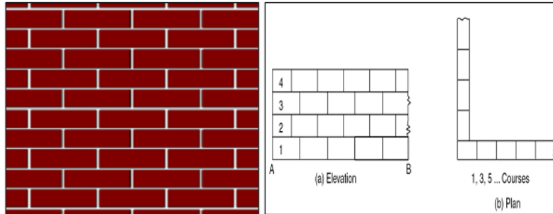
Figure-3.12. Stretcher Bond
